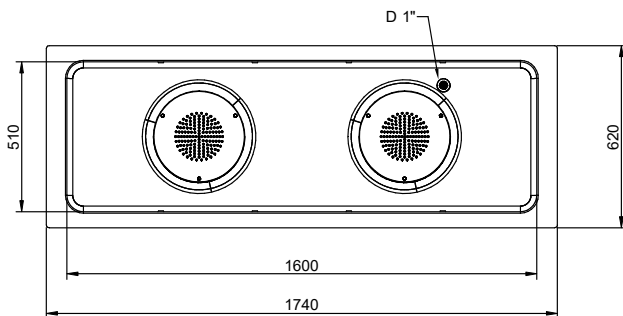
Boven aanzicht
